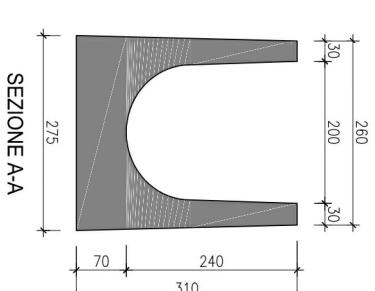
Canaletta di raccolta con griglia carrabile in progetto (vedi d.l.)
